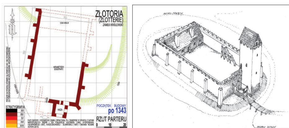
Rzut architektoniczny i hipotetyczna próba rekonstrukcji nadwodnego zamku Kazimierza III w Złotorii. Opracowanie i rysunek Piotr Zaniewski (2021)
